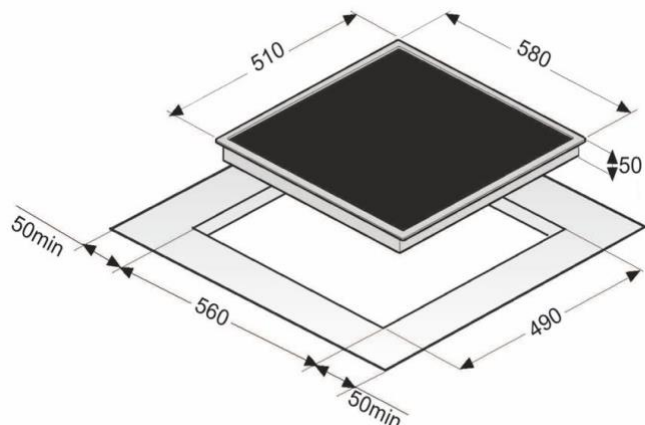
Diagrama de instalación
