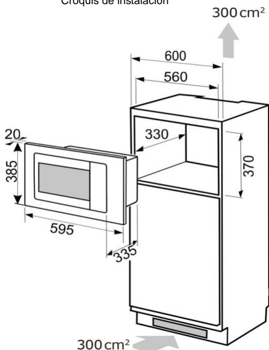
Croquis de instalación
